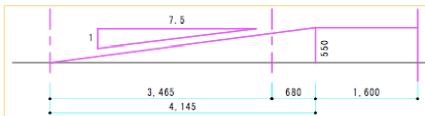
「車庫スロープ案 断面図」
